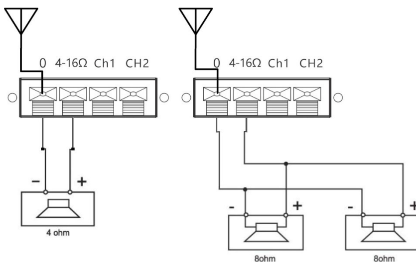
Schemat podłączeń głośników 4Ω i 8Ω
